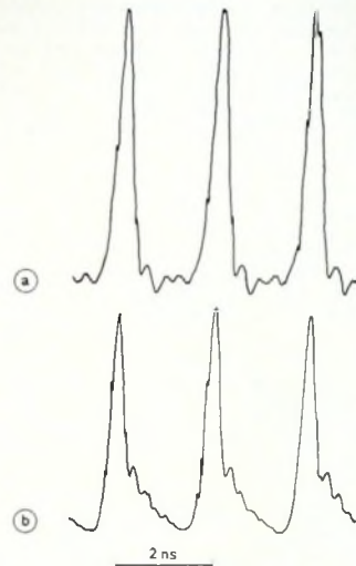
Bild 8. Modulation eines Doppelheterostruktur-Injektionslasers mit 500 Mbit/s; a) Steuerstrom, b) demoduliertes optisches Signal
