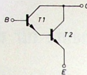
Bild 2. Innenschaltung der monolithischen Darlington-Transistoren von Texas Instruments
