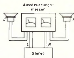
Bild 9. Anschluß des Geräts an eine Stereo-Anlage
