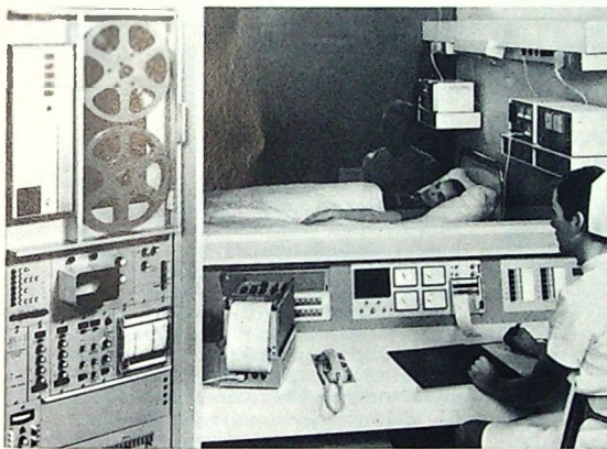
Bild 6. Analog-Magnetbandspeicher „Medi-tape AR“ für Vitalwerte mit Formanalysator für EKG und Elektrokardiograf zur Arrhythmieausschreibung (Siemens)
