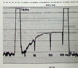
Bild 8. Schüttelresonanz des „M 15 E-Super“ mit Dual-1009-Tonarm
