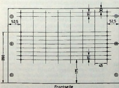
Bild 41. Bohrplan für Lüftungslöcher im Boden- und Deckelblech
