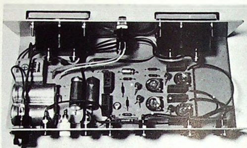
Bild 8. Blick in das fertig verdrahtete Gerät mit abgenommener Abdeckhaube
