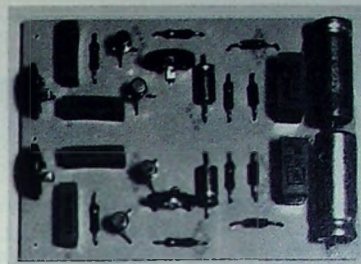
Bild 12. Platine und Bauelemente des Aussteuerungsmessers für Batteriebetrieb
