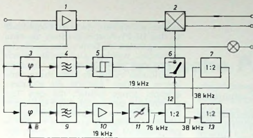
Bild 4. Blockschaltung des Stereo-Decoders MC 1310 P. 1 Eingangsverstärker, 2 Decoder, 3 Phasenkomparator zur Stereo-Identifikation, 4 Tiefpaß, 5 Schwellenwertschalter und Lampentreiber, 6 Stereo-Schalter, 7 Frequenzteiler, 8 Phasenkomparator zur Pilottonregenerierung, 9 Tiefpaß, 10 Gleichspannungsverstärker, 11 spannungsgesteuerter 76-kHz-Oszillator, 12 Frequenzteiler, 13 Frequenzteiler
