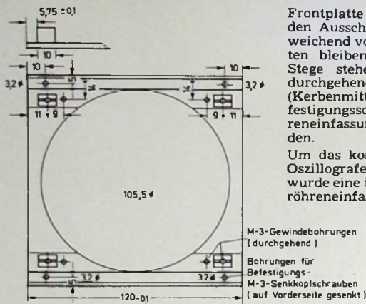
Bild 51. Frontplatte für Bildröhre
