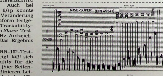
Bild 7. Frequenzgang des Nutzkanals und Übersprechen (ohne Terzfilter, Meßplatte DIN 45 541, Auflagekraft 1 p)
