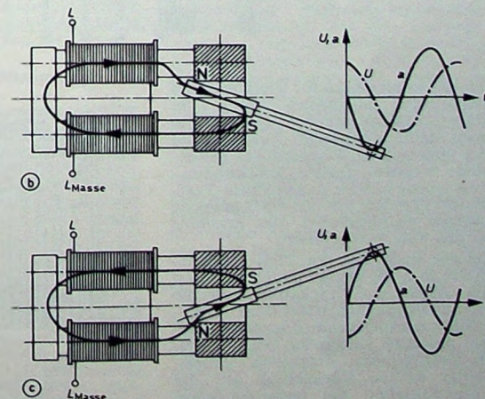
Bild 3. Wirkungsweise für einen Kanal des Tonabnehmers ( U = Spannung, a = Amplitude)
