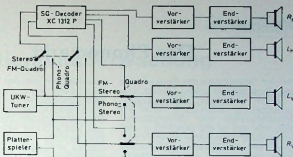
Bild 5. Blockschemata einer für Stereo- und Quadrophonie-Wiedergabe geeigneten Anlage mit dem SQ-Decoder XC 1312 P
