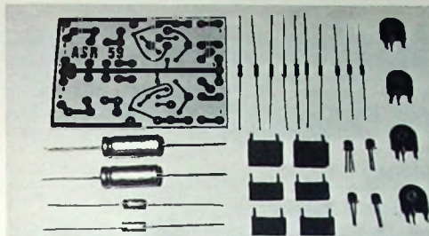
Bild 12. Platine und Bauelemente des Aussteuerungsmessers für Batteriebetrieb
