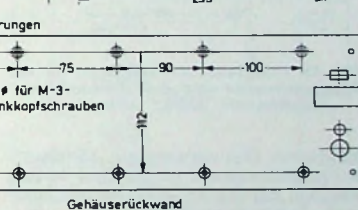
Bild 40. Gehäuserückwand
