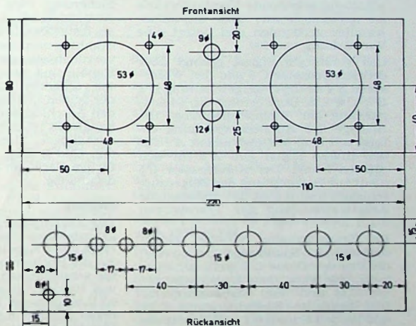
Bild 4. Bohrplan für die Front- und Rückwand
