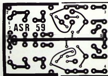
Bild 10. Printplatte des Aussteuerungsmessers für Batteriebetrieb (Maßstab 1:2)
