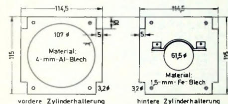
Bild 38. Montageteile für den Bildröhrenkomplex
