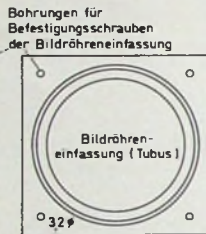
Bild 52. Raster und Einfassung (Tubus) der Bildröhre
