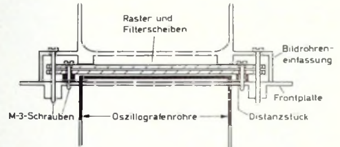
Bild 52. Raster und Einfassung (Tubus) der Bildröhre
