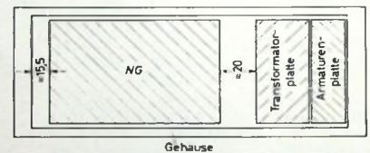
Bild 55. Abstände der befestigten Bauteile des hinteren Gehäuse Rahmens
