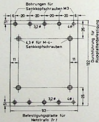
Bild 54. Hintere Armaturenplatte und Befestigungsplatte für Netztransformator Tr 1 (Material: 2-mm-Al-Blech)
