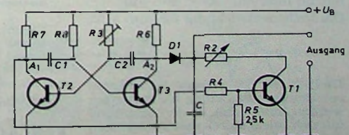
Bild 11. Praktische Schaltung zur Erzeugung einer e-Funktion
